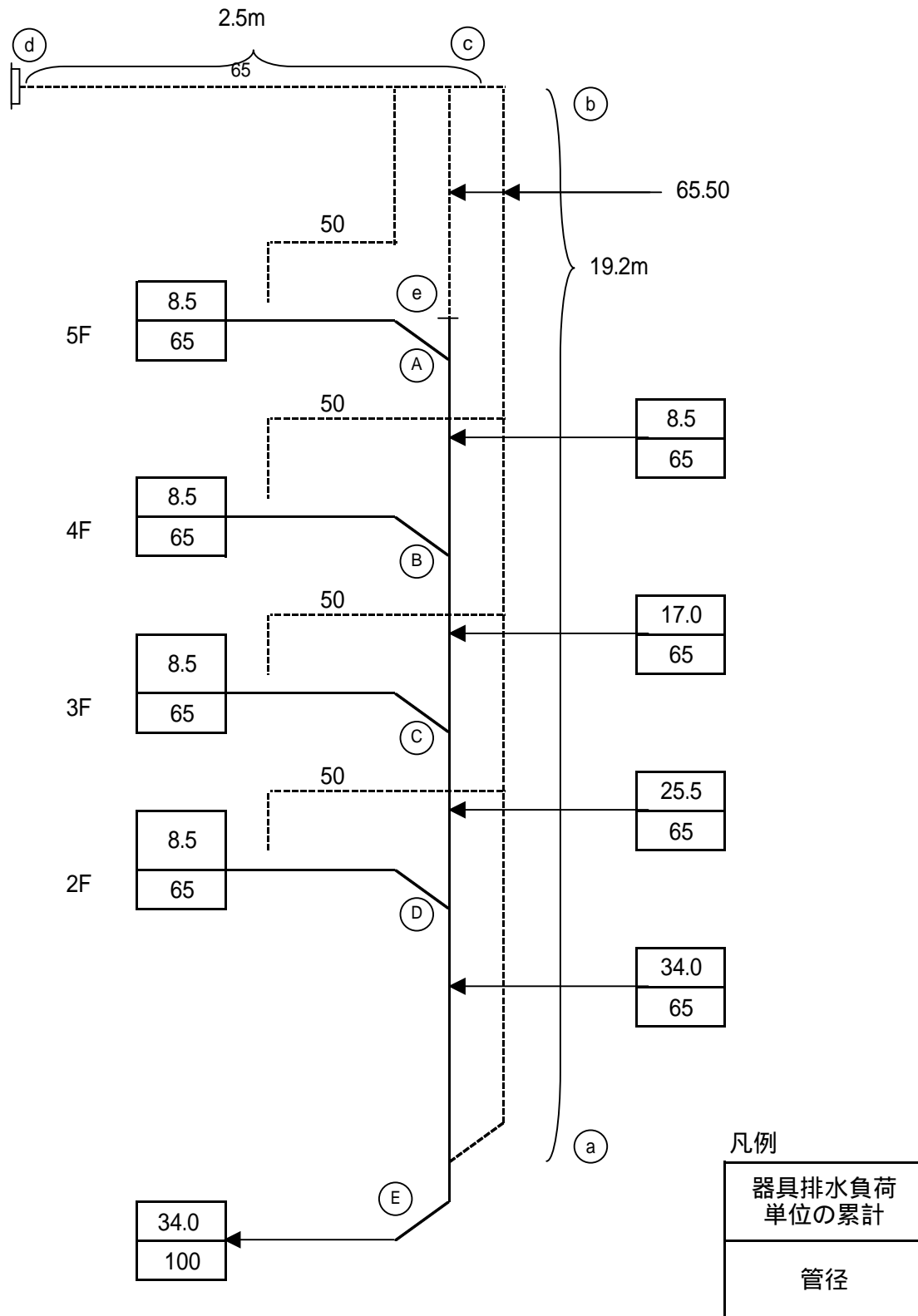
雑排水立て管系統図
